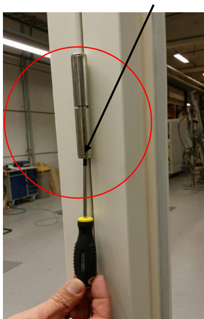
Høydejustering torx 15
