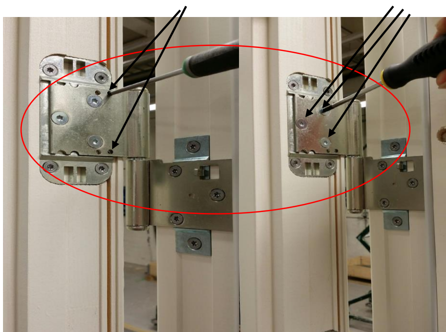
Justerskrue dørblad torx10. Låseskrue dørblad torx 20.
